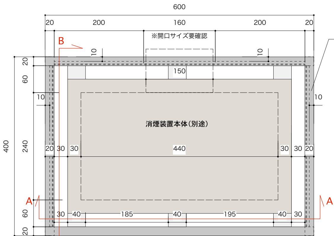
a 平面図
